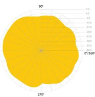
5GHz 2D 無線場形 @ 垂直方向
