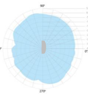
2.4GHz 2D 無線場形 @ 水平方向
