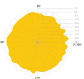
5GHz 2D 無線場形 @ 水平方向
