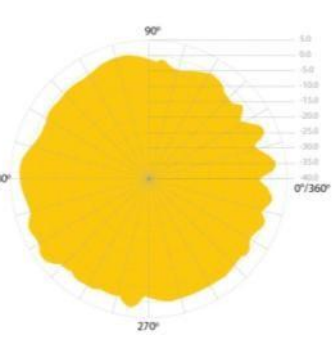
5GHz 2D 無線場形 @ 水平方向
